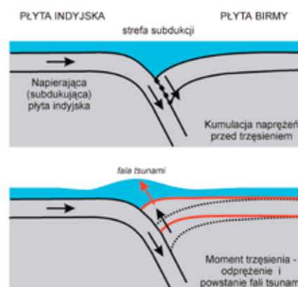
Rys. 4. Schemat mechanizmu powstawania trzęsienia ziemi i fali tsunami.
