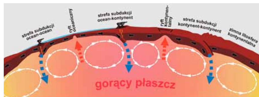
Rys. 3. Gorące wnętrze Ziemi napędza „maszynę ciepłą” – konwekcja w płaszczu Ziemi powoduje wynoszenie ciepłej materii w prądach wznoszących (strzałki czerwone) i powrót ochłodzonej materii do wnętrza Ziemi w prądach zstępujących (strzałki niebieskie). Ruch sztywnych płyt litosferycznych (strzałki czarne) prowadzi do ich kolizji w strefach subdukcji typu: ocean-ocean (np. Wyspy Mariańskie, Aleuty), ocean-kontynent (np. płyta Nazca i Ameryka Południowa), kontynent-kontynent (np. Indie i Azja – wypiętrzenie Tybetu i Himalajów). Układ komórek konwekcyjnych uzupełniają strefy ryftowe: oceaniczne (np. grzbiet śródatlantycki) i kontynentalne (ryft wschodnio-afrykański).
