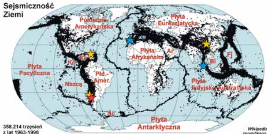
Rys. 2. Sejsmiczność Ziemi i podział na płyty litosferyczne. Niebieskie gwiazdki oznaczają lokalizację epicentrum trzęsienia z 1 listopada 1755, które spowodowało zniszczenie Lizbony oraz lokalizację epicentrum trzęsienia Sumatra – Andaman z 26 grudnia 2004. Czerwona gwiazdka oznacza lokalizację trzęsienia w Chile z 22 maja 1960 – największego trzęsienia w XX wieku, którego magnituda wynosiła M=9,5 . Pomarańczowe gwiazdki pokazują lokalizacje ostatnich katastrofalnych trzęsień w prowincji Sichuan (Chiny, 12 maja 2008, M=7,9 ), na Haiti (13 stycznia 2010, M=7,2 ) oraz trzęsienia w Chile (27 lutego 2010, M=8,8 ). Oznaczenia płyt litosferycznych: Ar – Arabska; Bi – Płyta Birmy; Fi – Filipińska; Ka – Karaibska; Ko – Kokosowa; Sc – Płyta Scotia.
